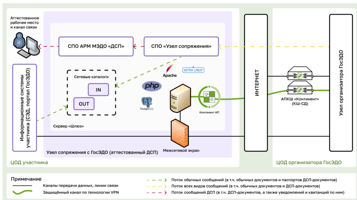
Рисунок 2. Типовая схема подключения СЭД участника к ГИС ГосЭДО с использованием модуля «Узел сопряжения» с обеспечением контура работы с ДСП документами в СПО АРМ МЭДО «ДСП» (Документооборот ДСП)
