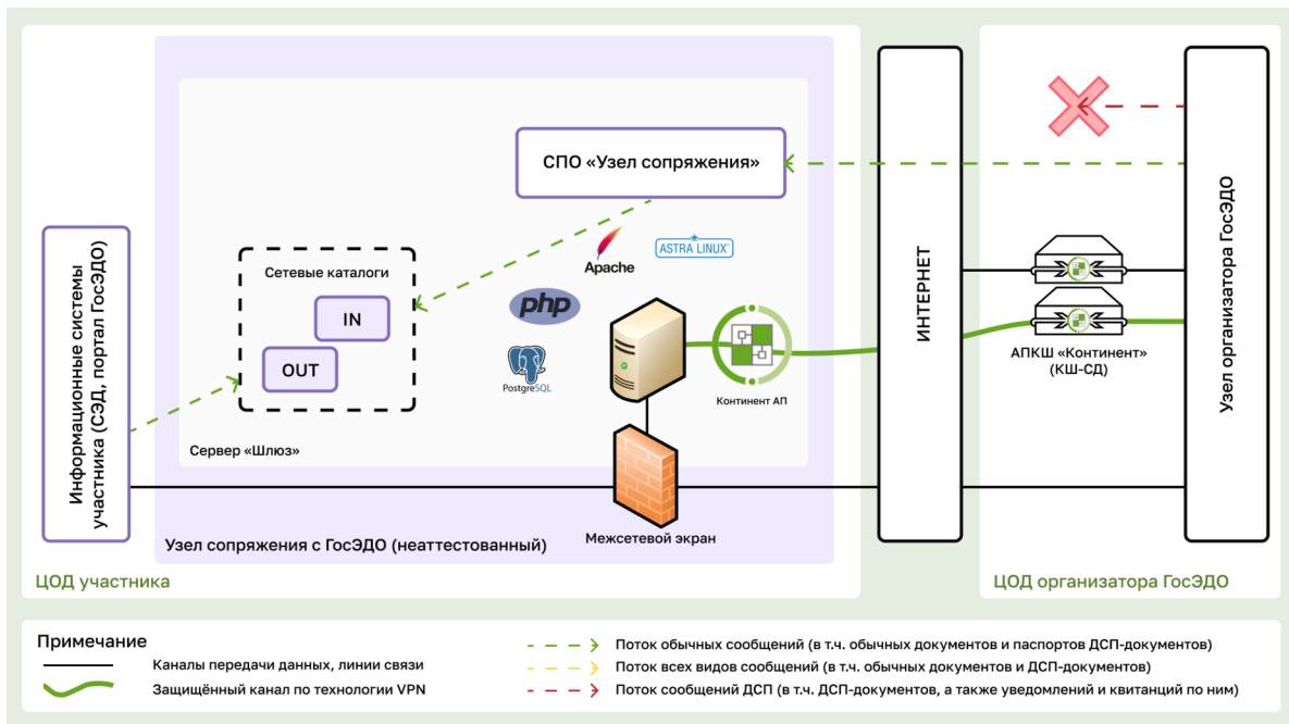
Рисунок 1. Типовая схема подключения СЭД участника к ГИС ГосЭДО с использованием модуля «Узел сопряжения» без организации отдельного контура работы с ДСП документами
