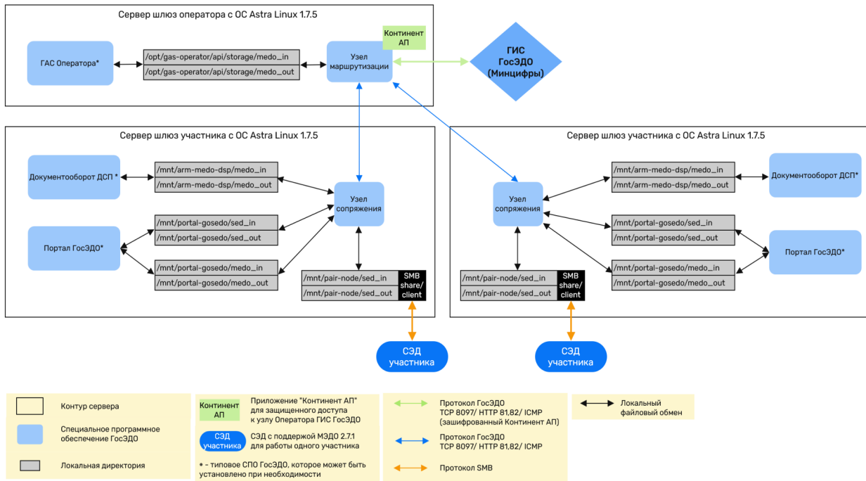
Рисунок 4. Типовая схема подключения оператора к ГИС ГосЭДО с использованием модуля «Узел маршрутизации», к которому подключены отдельные СЭД участников посредством модуля «Узел сопряжения», с обеспечением работы с документами ДСП у каждого участника
