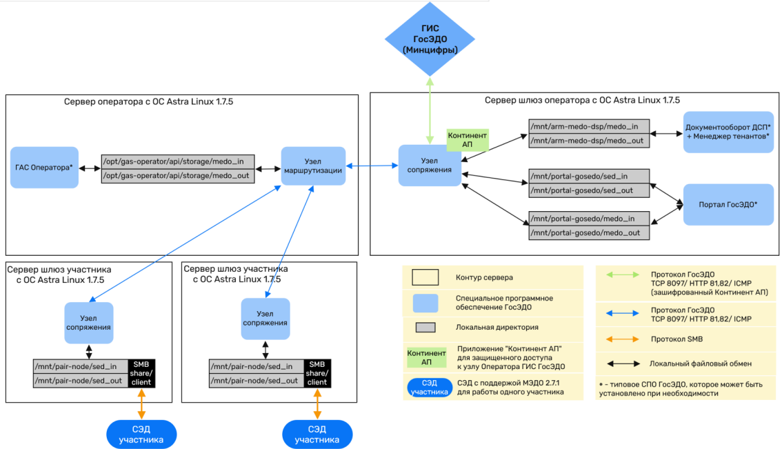
Схема 3.2 Оператор ГосЭДО (ГИС ГосЭДО, отдельные СЭД участников, ДСП с Менеджером тенантов)
