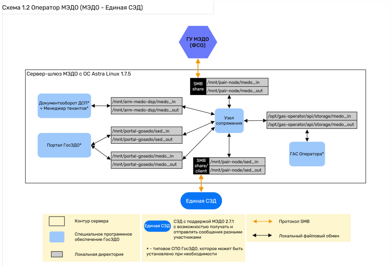
Рисунок 8. Типовая схема организации узла оператора МЭДО с использованием модуля «Узел сопряжения», единой СЭД для подключения участников и комплекта СПО для работы участников с документами ДСП на узле оператора
