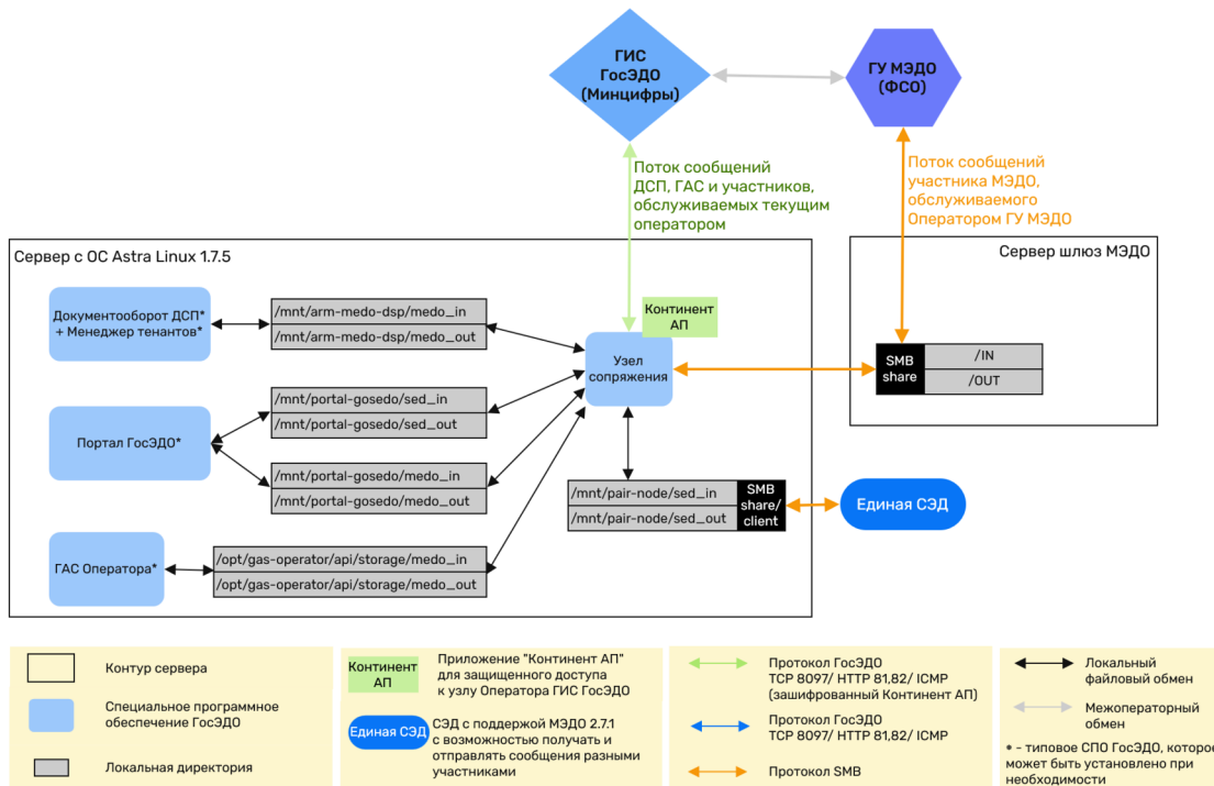
Рисунок 6. Комбинированная схема подключения оператора к ГИС ГосЭДО с использованием модуля «Узел сопряжения», установкой комплекта СПО для работы участников с ДСП документами на узле оператора и организацией потока сообщений участника МЭДО, обслуживаемого «Оператором ГУ МЭДО»
