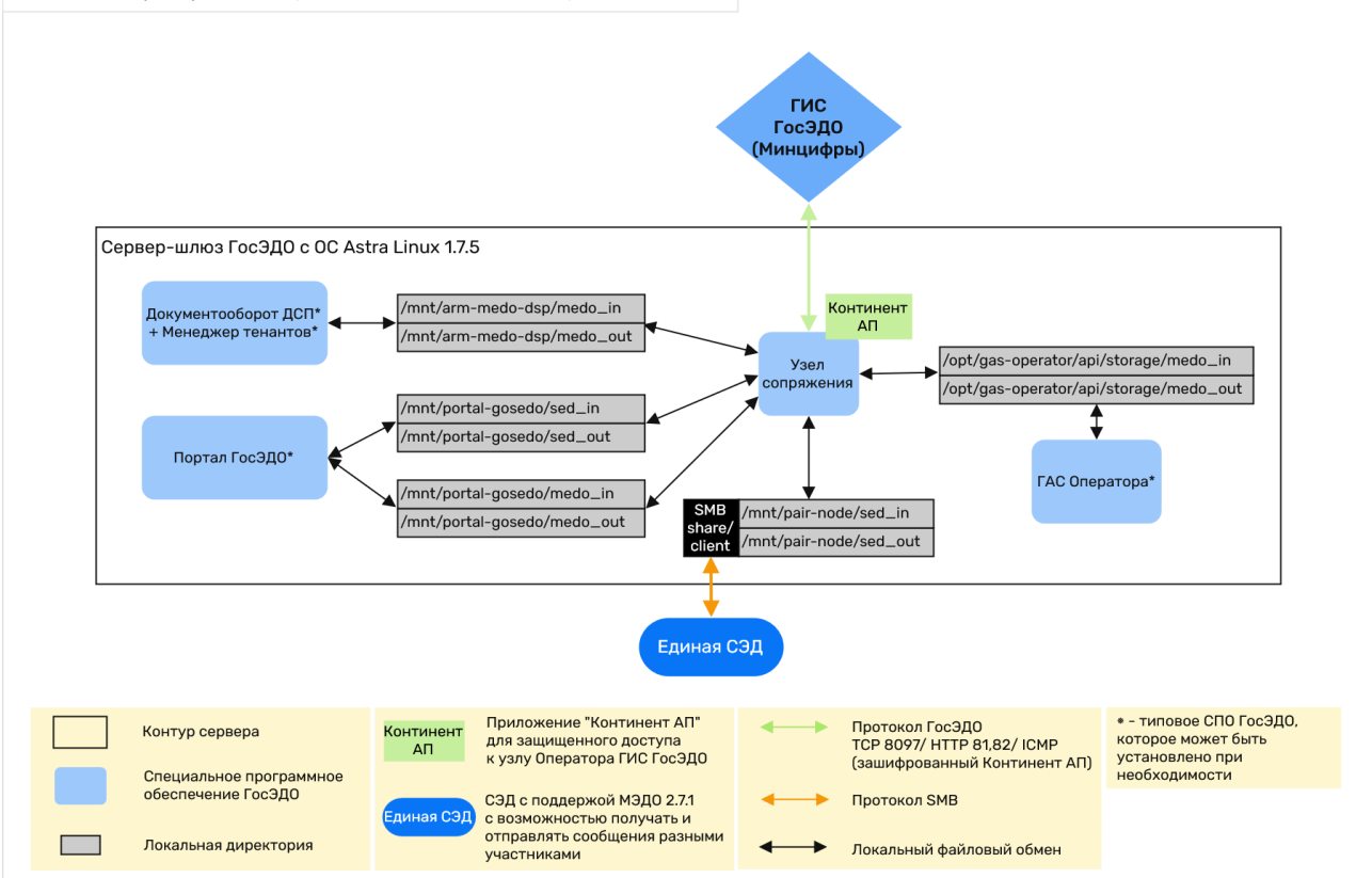
Рисунок 3. Типовая схема подключения оператора к ГИС ГосЭДО с использованием модуля «Узел сопряжения», единой СЭД для подключения участников и комплекта СПО для работы участников с документами ДСП
