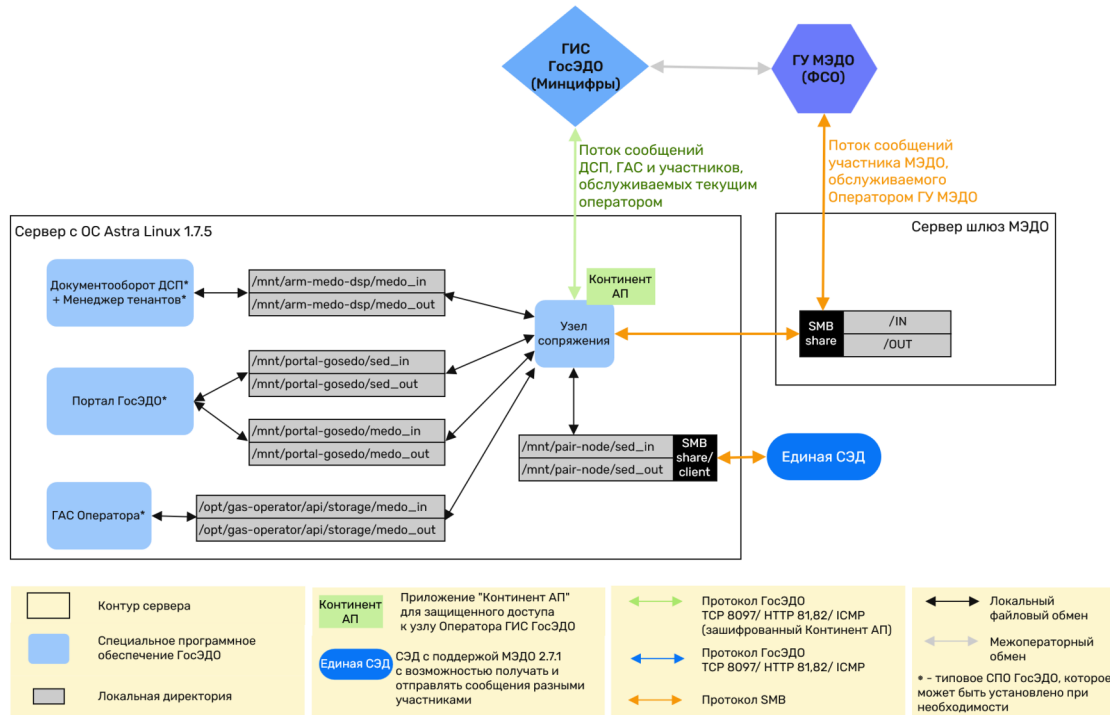
Схема 2.1 Оператор ГосЭДО, СЭД МЭДО (Оператор ГосЭДО, Единая СЭД, отдельный поток сообщений участника МЭДО)
