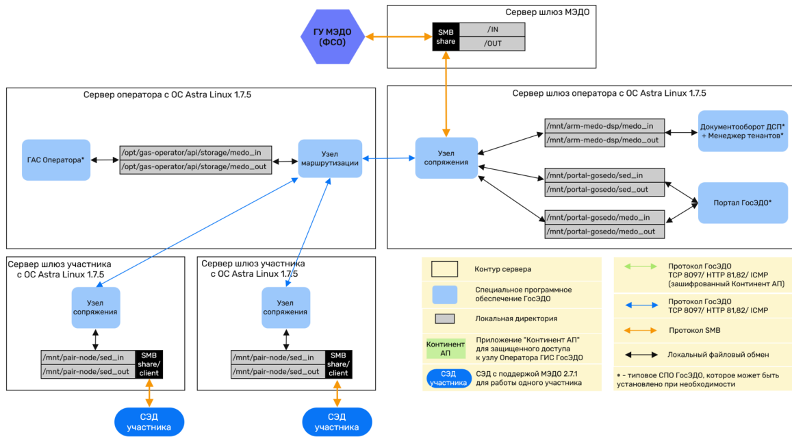
Рисунок 10. Типовая схема организации узла оператора МЭДО с использованием модулей «Узел сопряжения» и «Узел маршрутизации», с установкой комплекта СПО для работы участников с ДСП документами на узле оператора, отдельные СЭД участников подключены к оператору с использованием модуля «Узел сопряжения»
