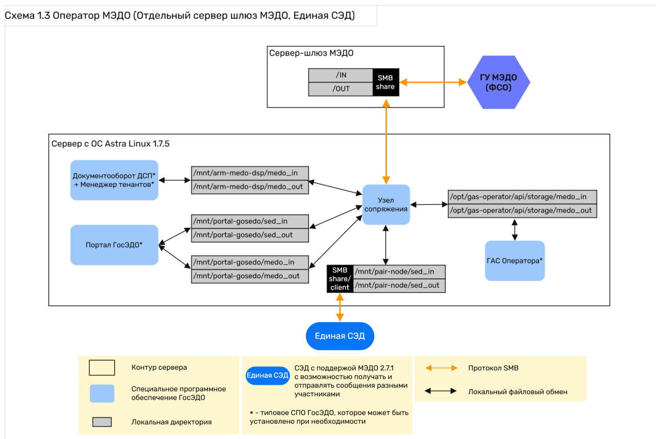
Рисунок 9. Типовая схема организации узла оператора МЭДО с использованием модуля «Узел сопряжения», единой СЭД для подключения участников и комплекта СПО для работы участников с документами ДСП на узле оператора (шлюз МЭДО на отдельном сервере)
