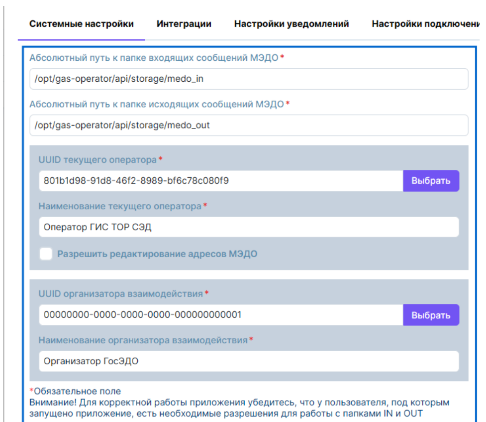
Рисунок 2.15. Набор полей выбранной вкладки
