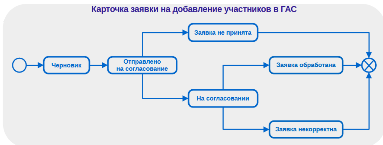
Рисунок 5.16.1. Схема движения карточки заявки на добавление участников в ГАС по статусам
