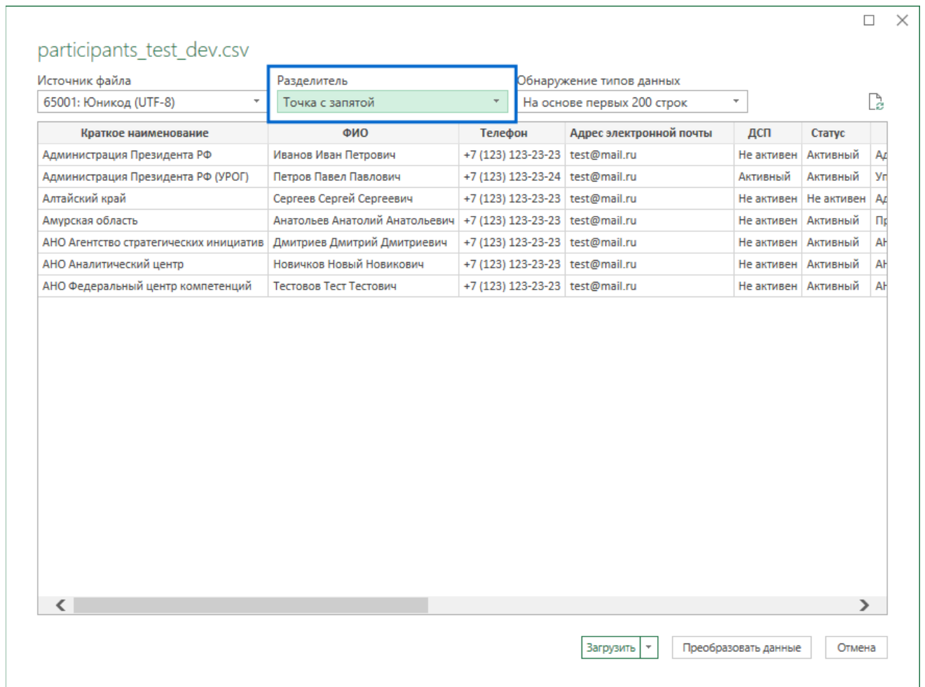
Рисунок 7. Значение в поле «Разделитель»
