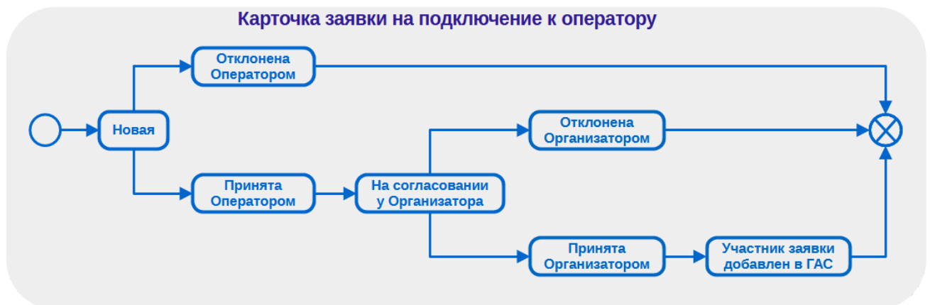
Рисунок 5.6.1. Схема движения карточки заявки на подключение к оператору по статусам
