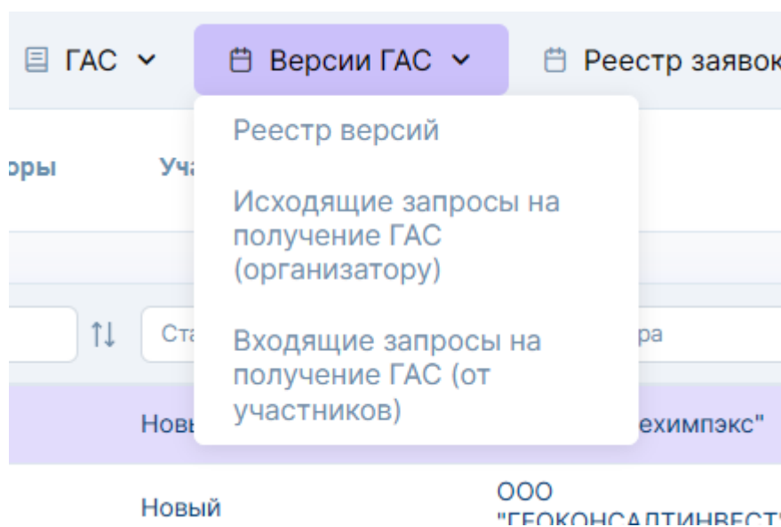
Рисунок 4.1. Пункты списка «Версии ГАС» главного меню Программы
