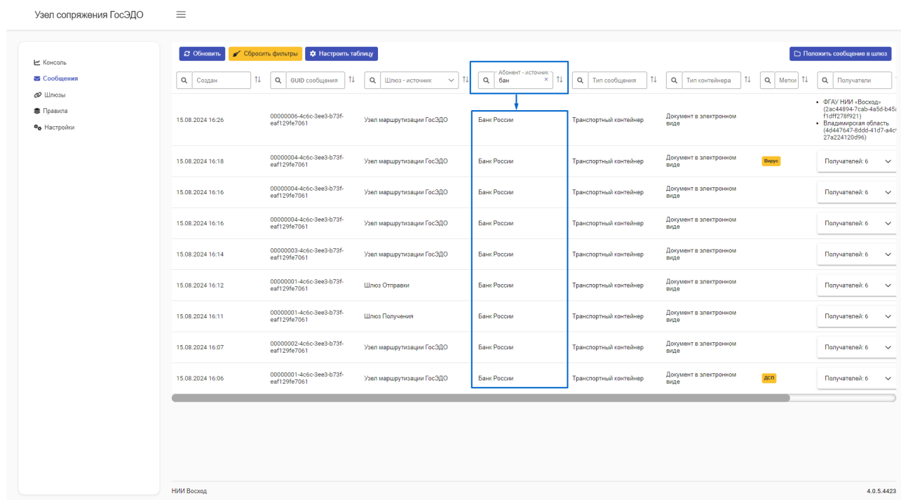
Рисунок 4.11. Результат фильтрации по текстовому полю
