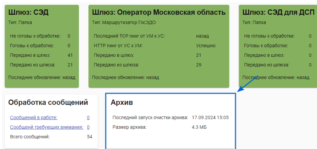
Рисунок 8.16. Блок «Архив» консоли мониторинга
