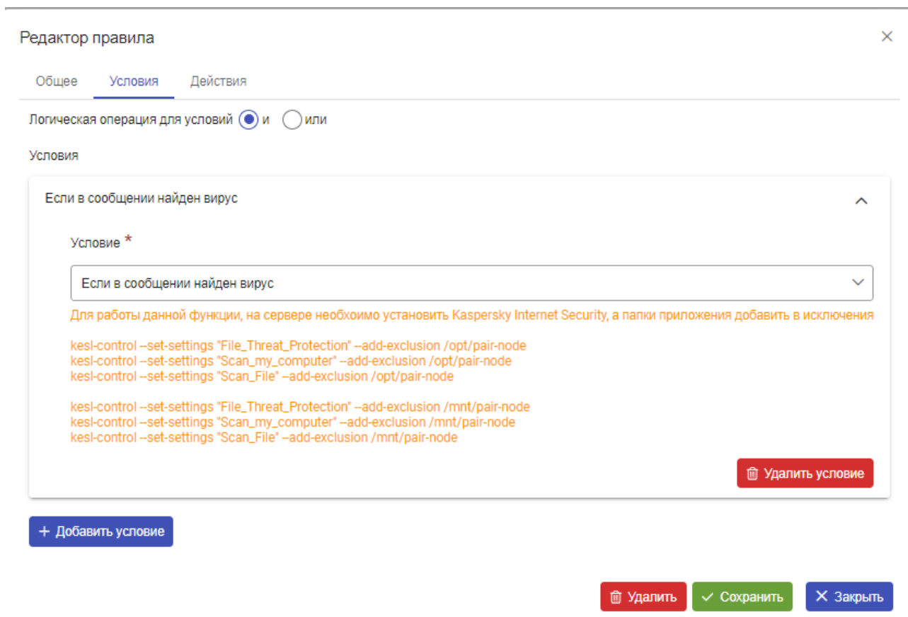
Рисунок 6.19. Условие «Если в сообщении найден вирус»
